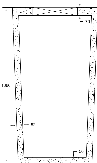
LID PLAN VIEW SCALE: 1:15
