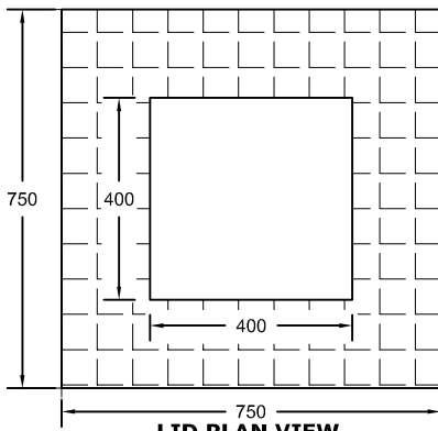
LID PLAN VIEW SCALE: 1:15
